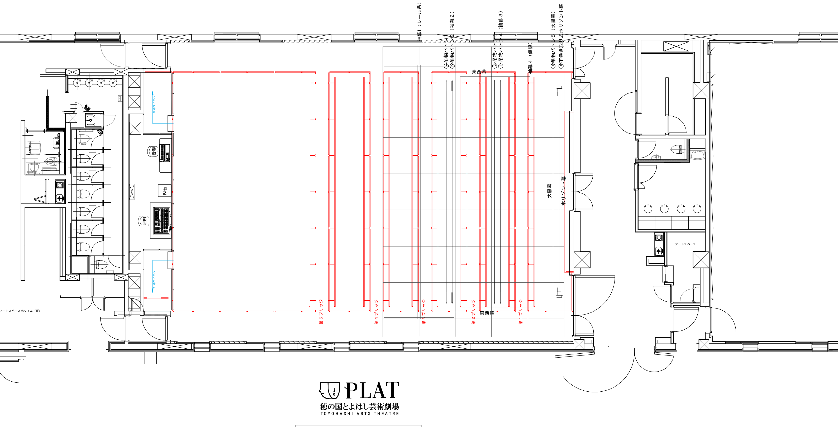
アートスペース 平面図 1/100 (A3)
